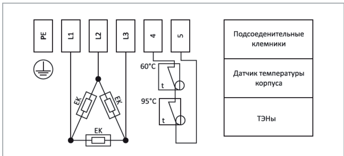
Электрическая схема подключения электронагревателей (рис. 19)
