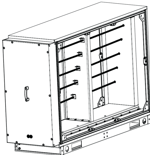
Электронагреватель (рис. 18)
